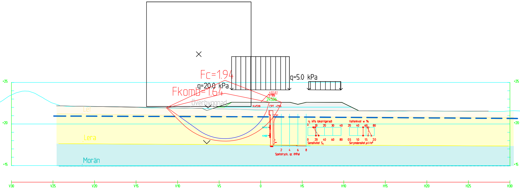
TVÄRSEKTION 1/100 1 100
